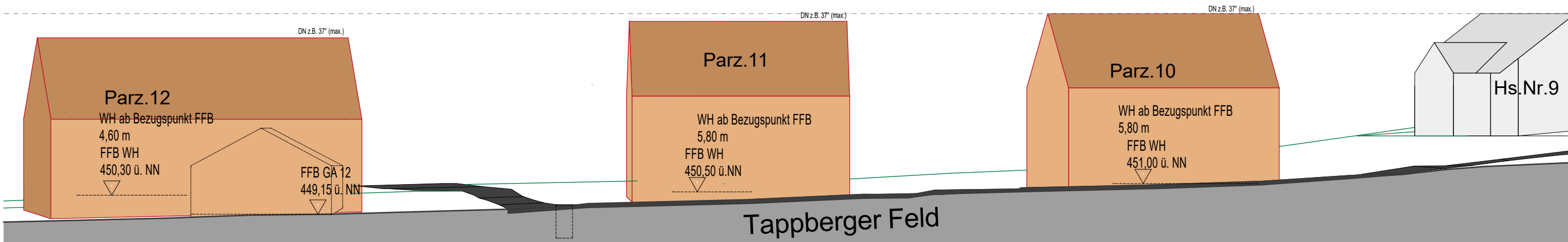
Schnitt: Süd - Nord M 1:250
